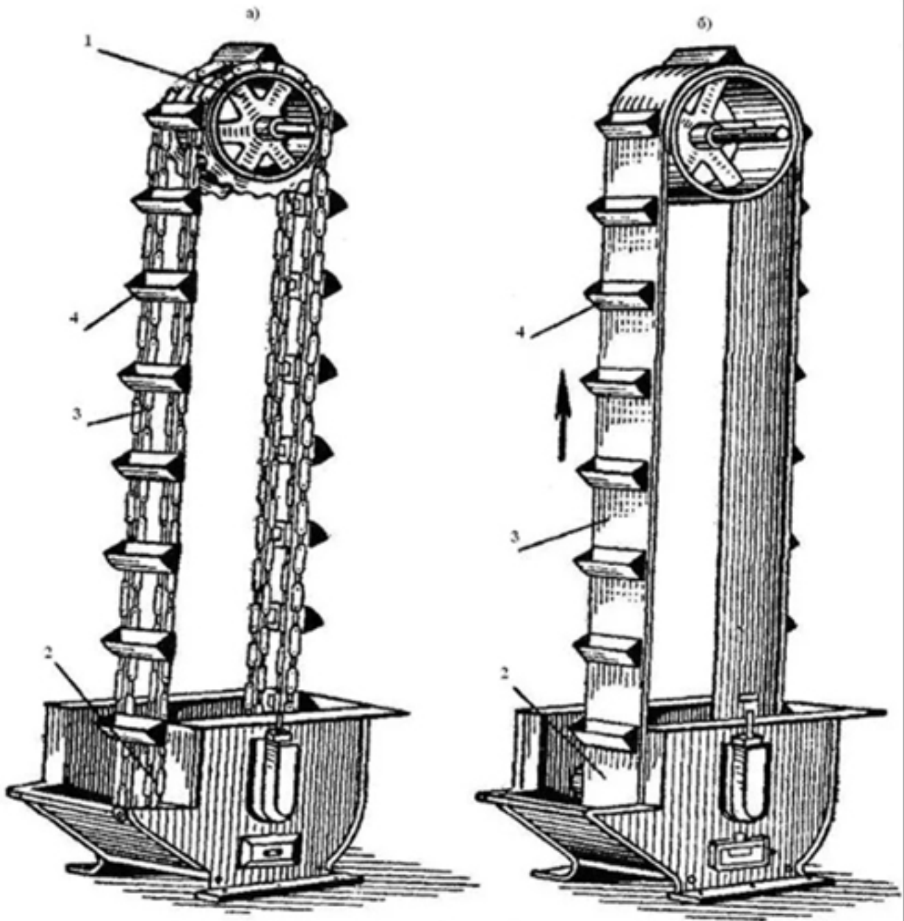
Рис. 5.27 Схемы ковшовых элеваторов: а — цепной; б — ленточный.
