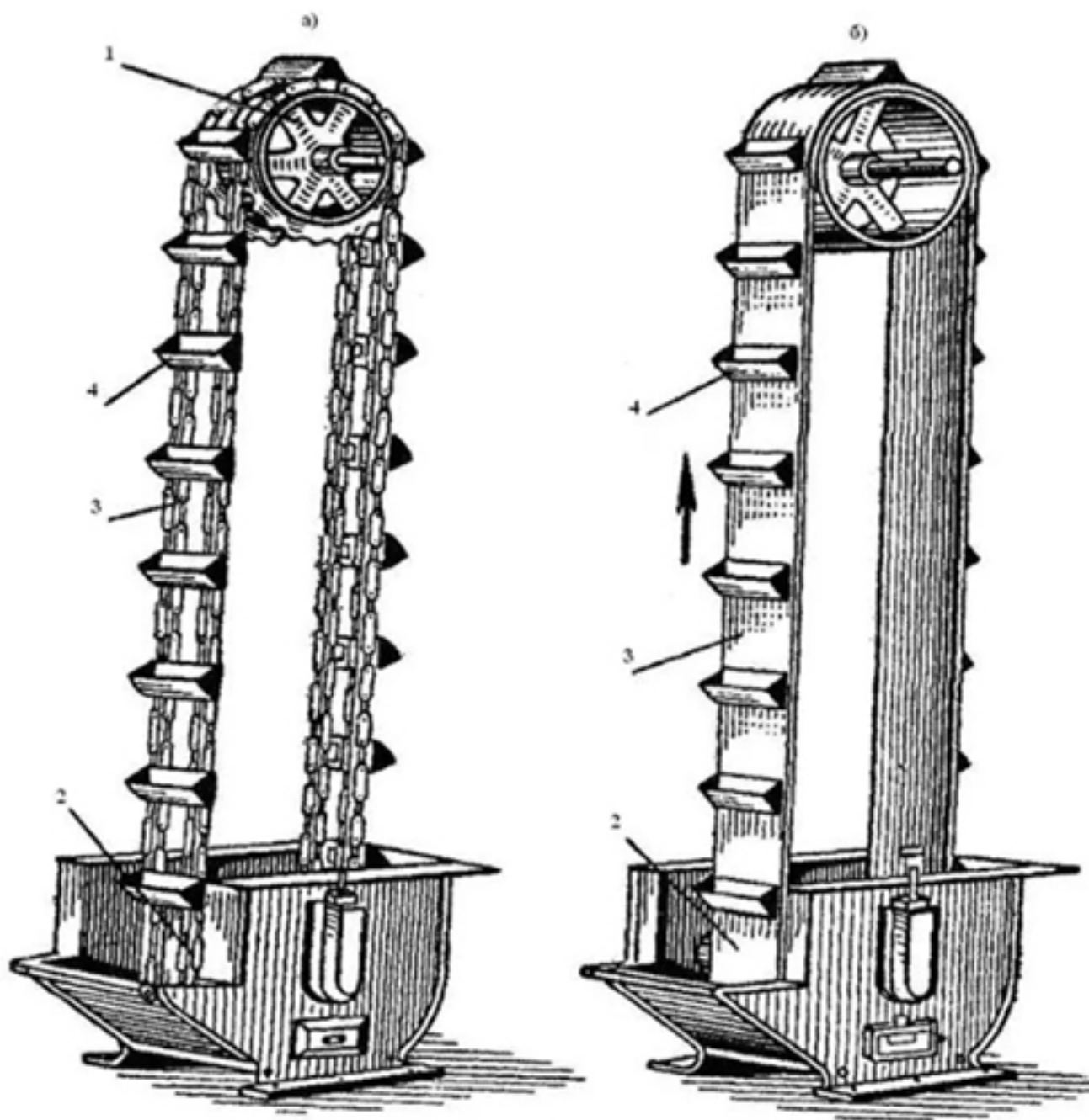
Рис. 5.27 Схемы ковшовых элеваторов: а — цепной; б — ленточный.
